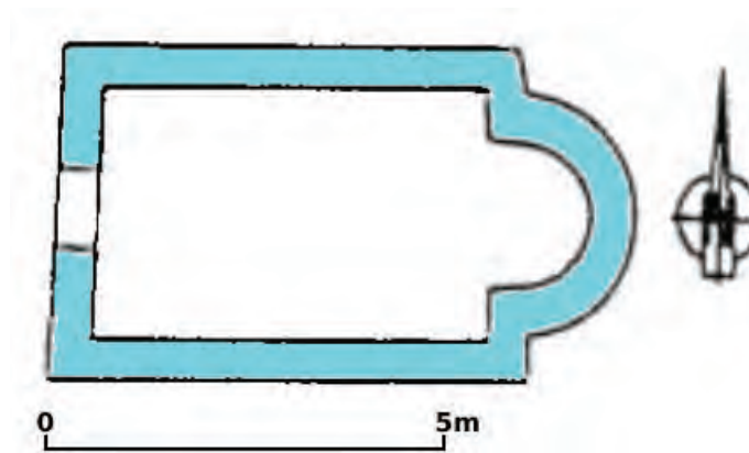
Slika 47 — Tlocrt ranokršćanske crkve sv. Tudora kod Nerežišća (prema: Chevalier 1995b, Pl. XLIX, obradio V. Barbarić)
