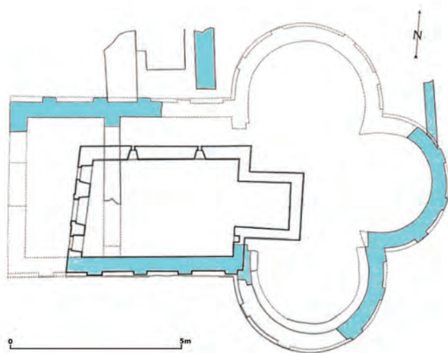
Slika 49 — Ranokršćanska crkva sv. Ivana u Sutivanu (prema: Belamarić et al. 1994, 66, obradio V. Barbarić)
