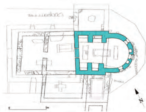
Slika 76 — Sv. Stjepan u Stipanskoj luci, crkva benediktinskoga samostana (prema: Bužančić 2000, 112, obradio V. Barbarić)
