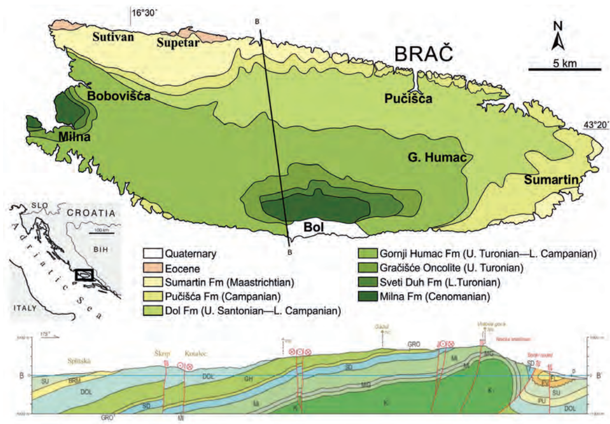
Slika 1 — Karta geoloških formacija i geološki presjek otoka Brača (prema: Schlagintweit, Cvetko Tešović 2017, Fig. 1 i Korbar et al. 2016, doradio V. Barbarić)
