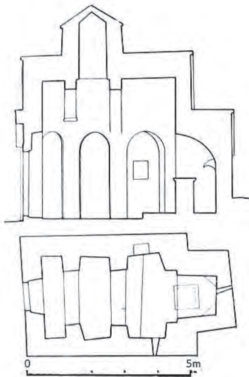
Slika 65 — Presjek i tlocrt Sv. Nikole kod Selaca (prema: Domančić 1960, 114, obradio V. Barbarić)
