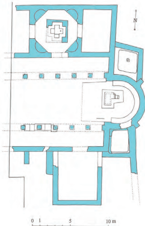
Slika 38 — Tlocrt ranokršćanskoga kompleksa u Postirama (prema: Belamarić et al. 1994, 45, doradio V. Barbarić)
