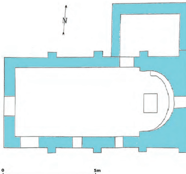
Slika 45 — Tlocrt ranokršćanske crkve sv. Jadre kod Škripa (prema: Belamarić et al. 1994, 75, obradio V. Barbarić)
