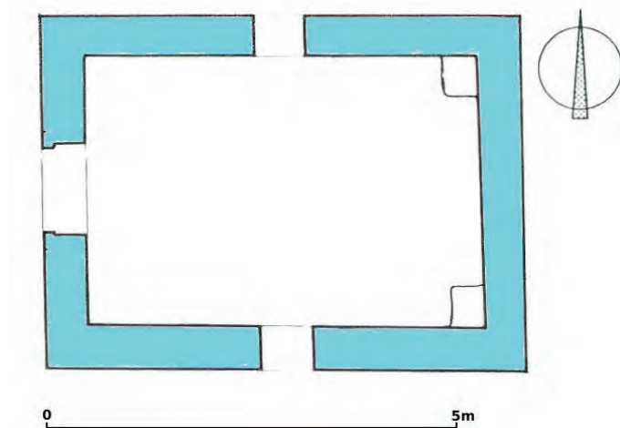
Slika 48 — Tlocrt ranokršćanske faze crkve sv. Ivana u Bolu (prema: Bužančić, 1991, 31, obradio V. Barbarić)
