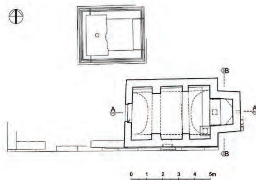
Slika 93 — Tlocrt Sv. Ilije, rimskog mauzoleja i ostataka arhitekture (prema: Fisković, Fisković 2011, 13.)
