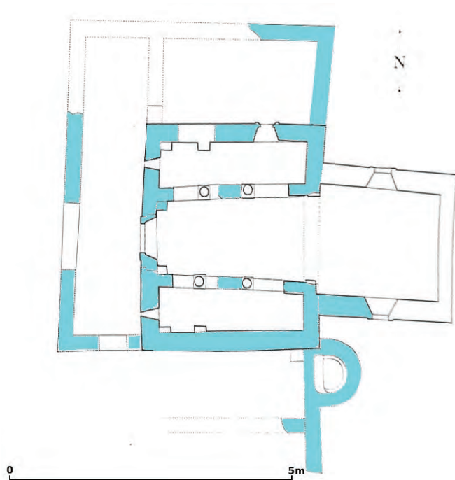
Slika 46 — Tlocrt ranokršćanske faze crkve sv. Duha u Škripu (prema: Belamarić et al. 1994, 81, obradio V. Barbarić)
