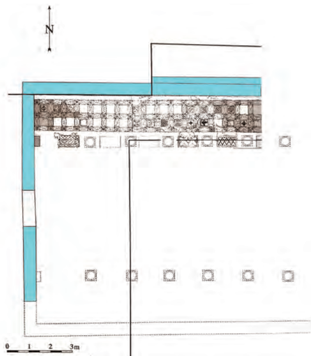
Slika 50 — Tlocrt istražene površine s rekonstrukcijom istočnoga dijela ranokršćanske bazilike u Supetru (prema: Belamarić et al. 1994, 62, obradio V. Barbarić)
