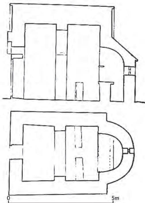
Slika 104 — Sv. Marija, tlocrt i presjek (prema: Domančić 1960, 126.)
