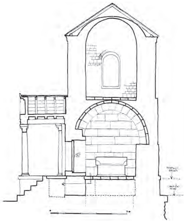
Slika 30 — Mauzolej/heroon u Škripu (prema: Faber, Nikolanci 1985, Slika 2.)
